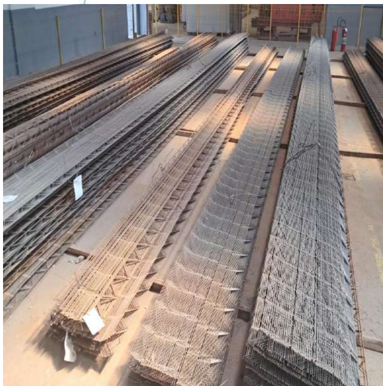
Foto 040: Treliças
